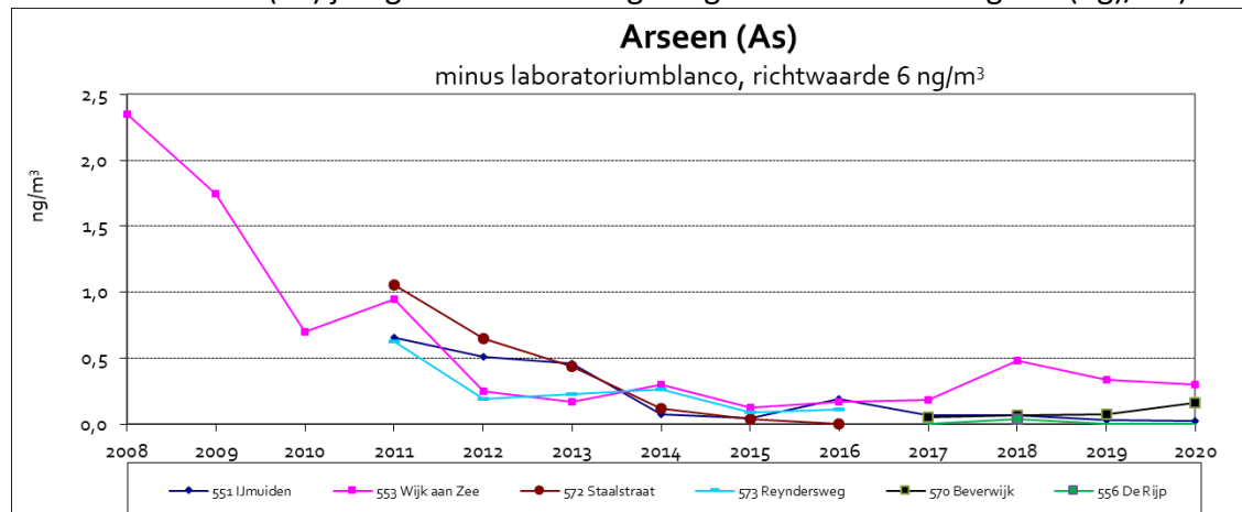
Grafiek 2: Arseen (As) jaargemiddelden omgeving Tata Steel in nanogram (ng)/m 3
