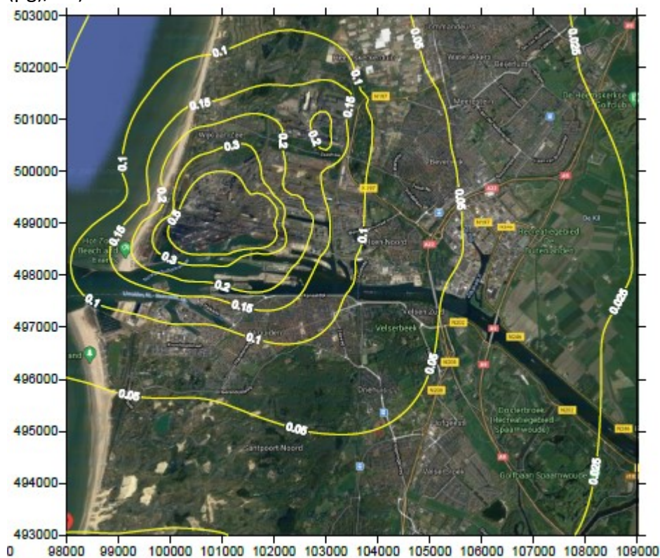
Tata Steel berekende immissiecontour 3 bij bepaalde emissie: Arseen in microgram (μg)/m 3
