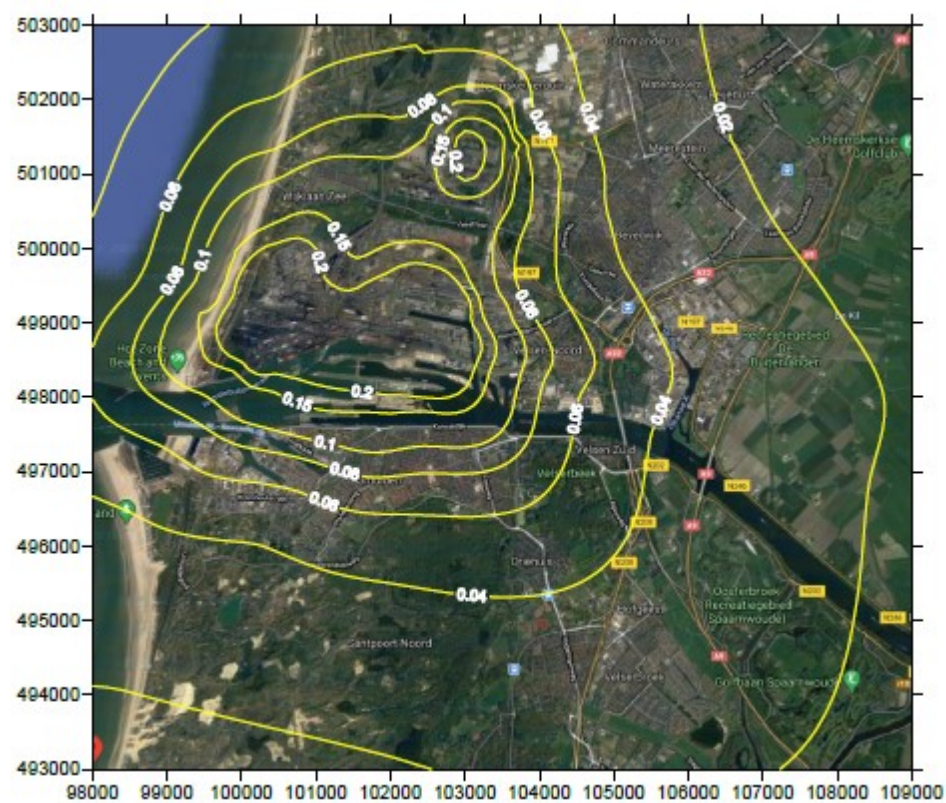
Tata Steel berekende immissiecontour 1 bij bepaalde emissie: Benzo(a)pyreen (BaP) in nanogram (ng)/m 3
