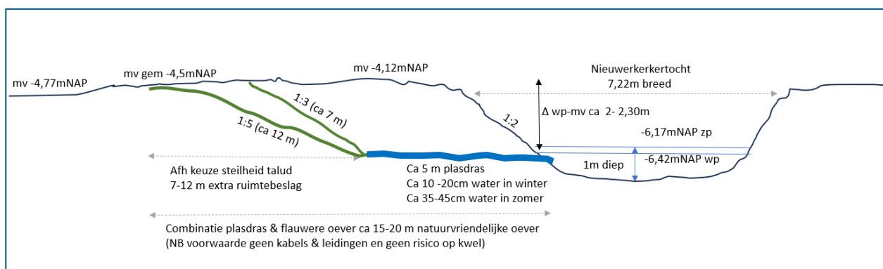
Figuur 4-9 Schets ontwerpprincipe plasdrasberm ter hoogte van Nieuwerkerkertocht. Afmetingen nader uit te werken.
